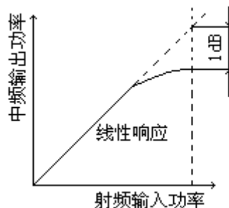
图 1 1dB 压缩点
